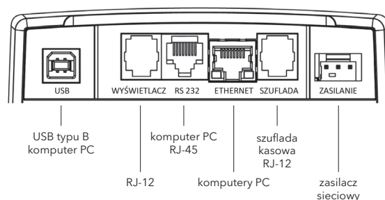
Złącza interfejsów w podstawie drukarki
